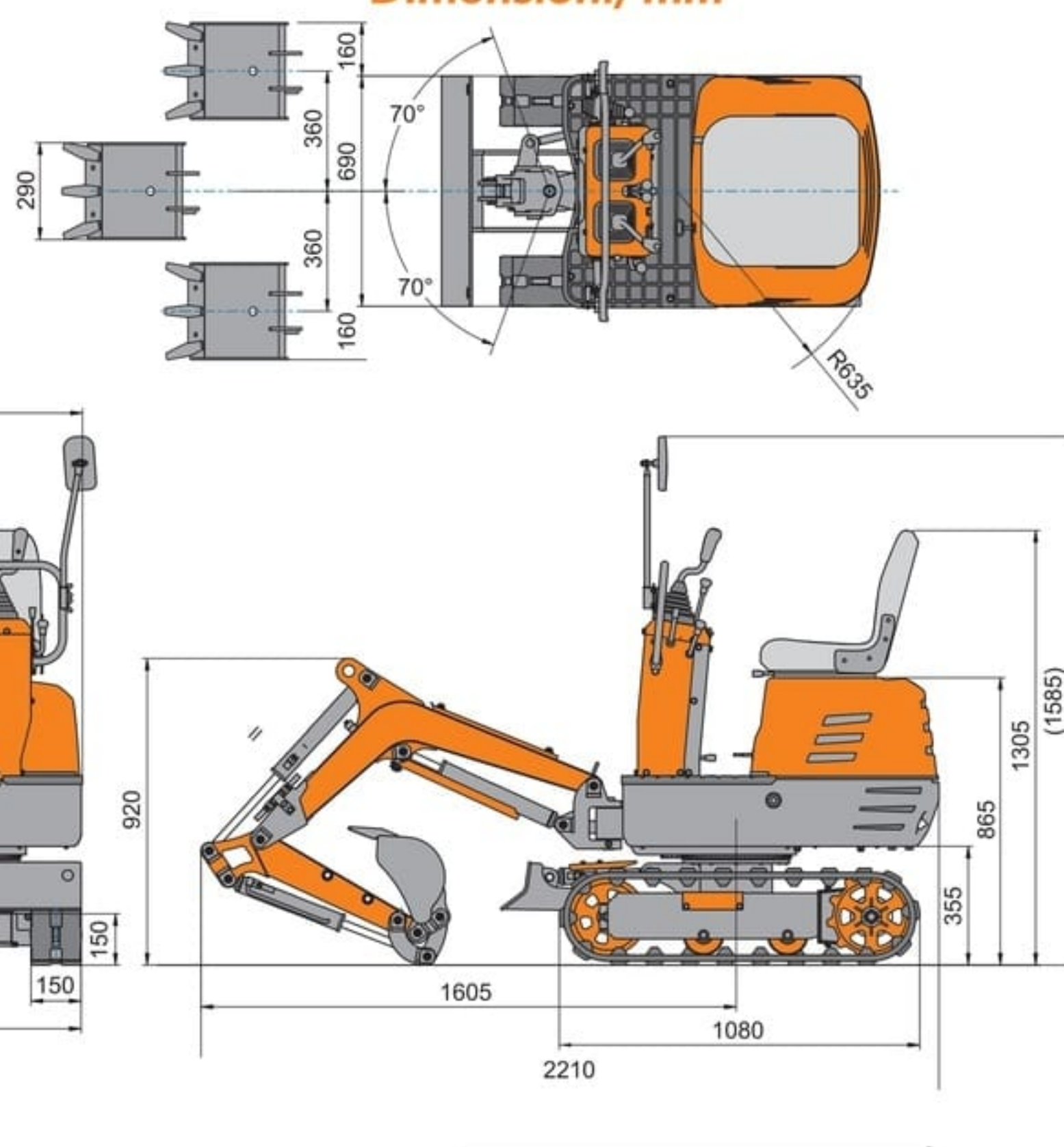
Dimensioni, mm
